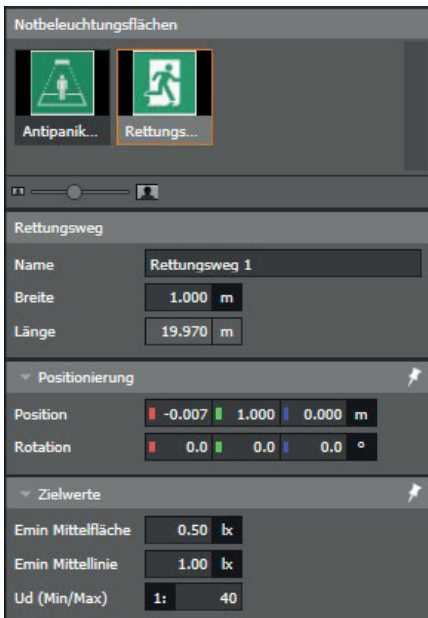
Bild 11.3: Konfiguration von Rettungswegen / Fluchtwegen und deren Beleuchtungsstärken
