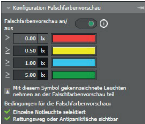
Bild 11.11: Kombination von Beleuchtungsstärken und Farben
