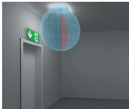
Bild 3.5b: beleuchtetes / außenbeleuchtetes Sicherheitszeichen
