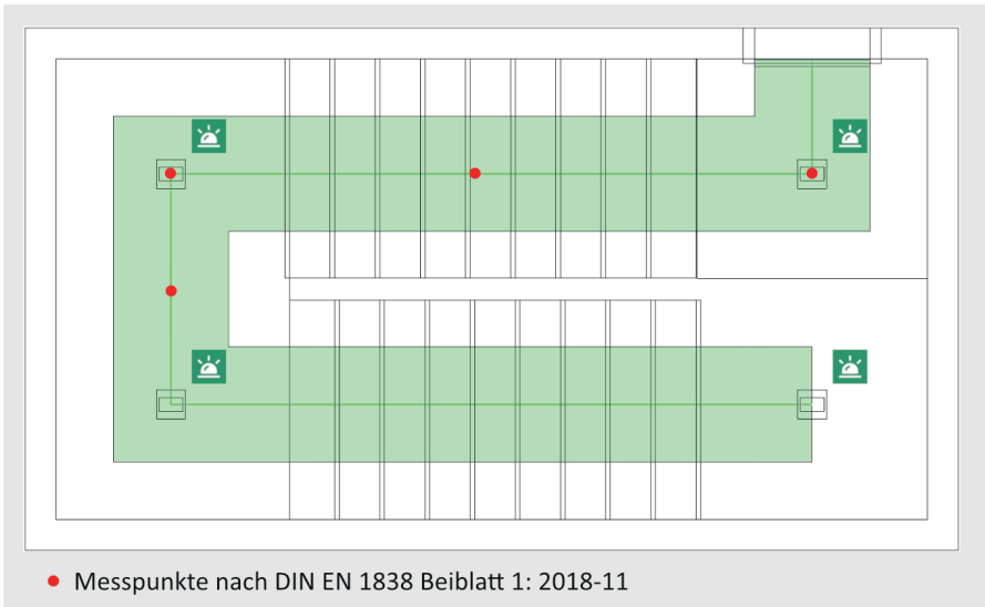
Bild 9.2b: Messpunkte für die Erstmessung in Treppenhallen in Anlehnung an die DIN EN 1838 Beiblatt 1: 2018-11
